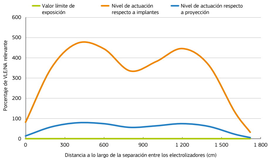
Figura 3.9. Variación de la densidad de flujo magnético estático a lo largo de la separación entre dos electrolizadores
