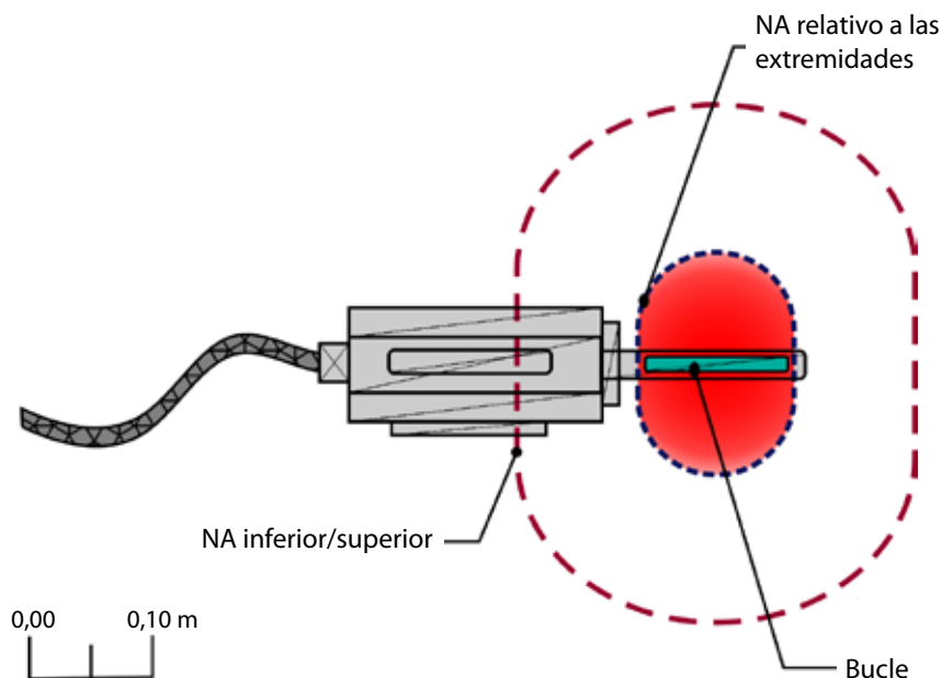
Figura 6.8. Vista en planta que muestra los contornos dentro de los cuales podrían superarse el nivel de actuación relativo a las extremidades (azul) y los niveles inferior/superior (rojo) en torno a la pistola de «tipo C» del taller de reparación cuando se equipa con un brazo de 160 mm
