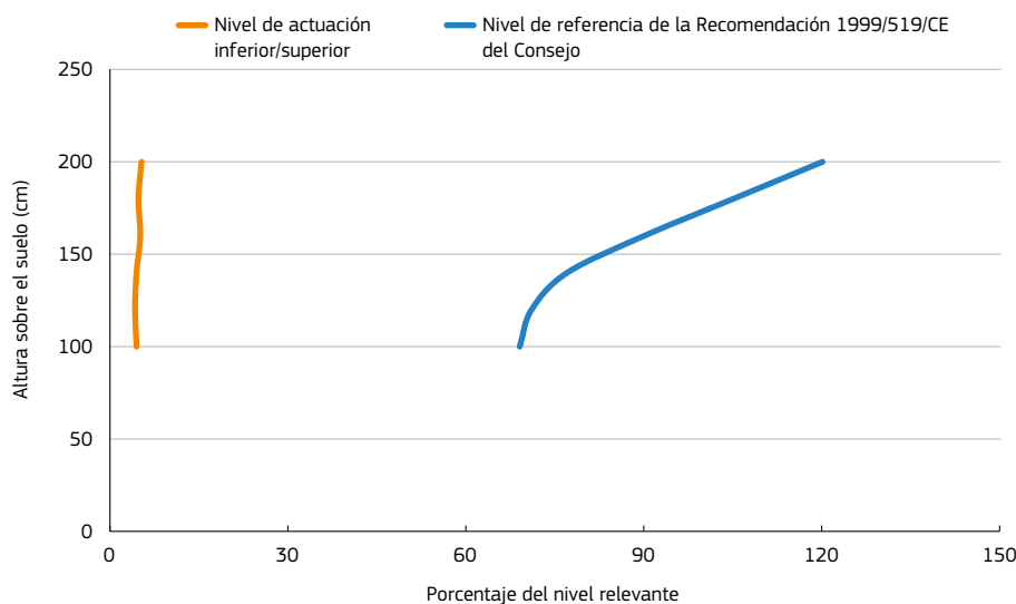
Figura 3.15. Variación de la densidad de flujo magnético variable con el tiempo de 300 Hz con la altura bajo el aislante de CC de la barra ómnibus
